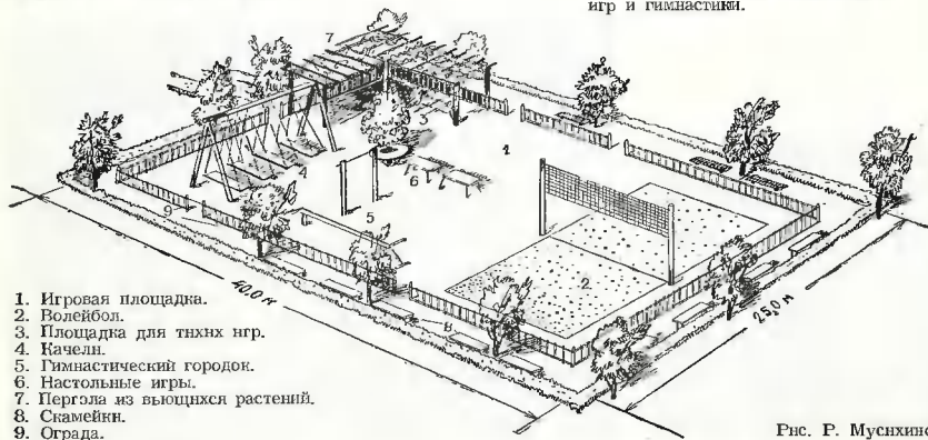
Рис. 4. Пример устройства детской площадки для спортивных игр и гимнастики.
